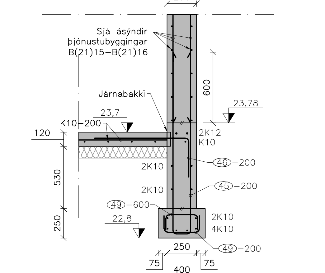
Z B(12)01 B(12)02 Sökkull i mätlinu 2 Mkv: 1:20
