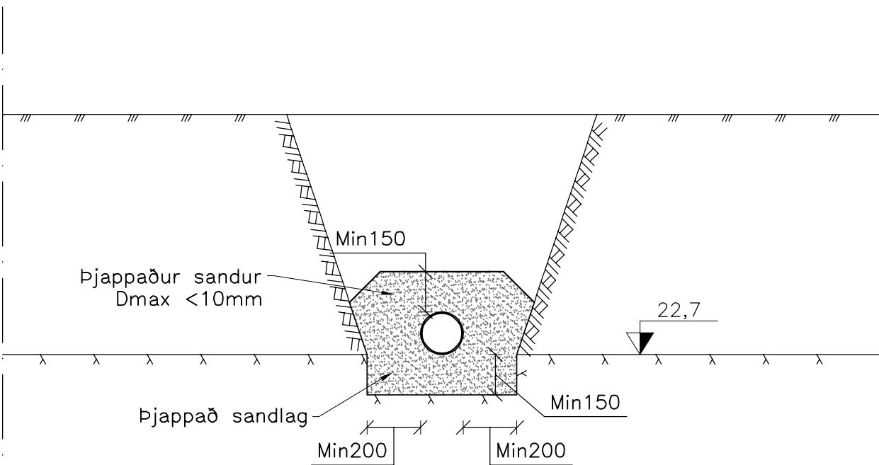
S9 J(11)05 Lagnaskurður Mkv: 1:20
