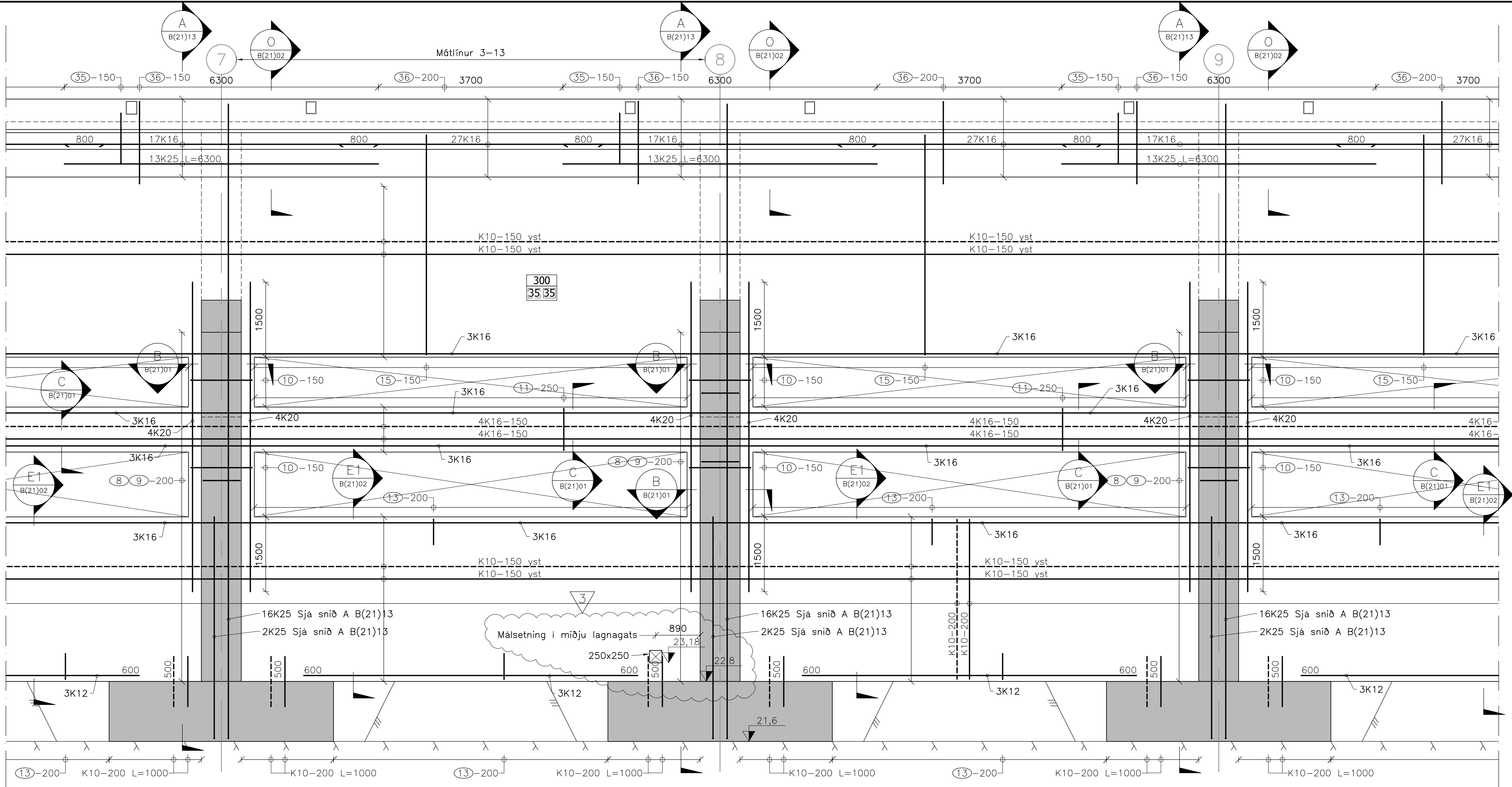
Veggur í mátlínu K Mkv: 1:50
