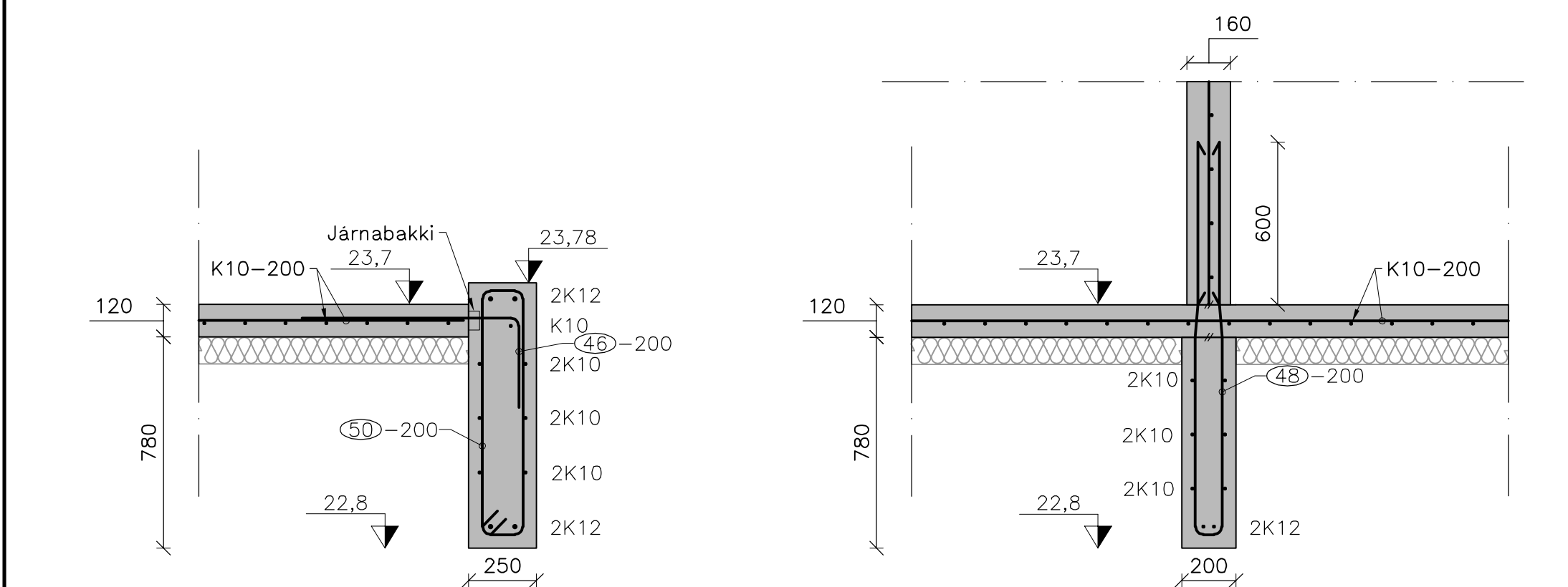
T B(12)02 B(12)03 B(13)01 B(21)01 B(21)15 Snið i sökkul þjónustubyggingar Mkv: 1:20
