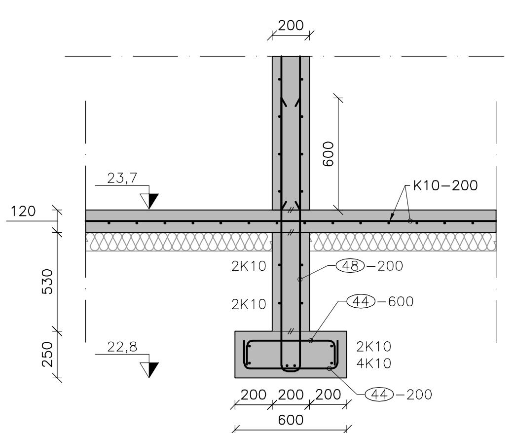
V B(12)02 B(12)03 B(21)16 Snið i sökkul þjónustubyggingar Mkv: 1:20
