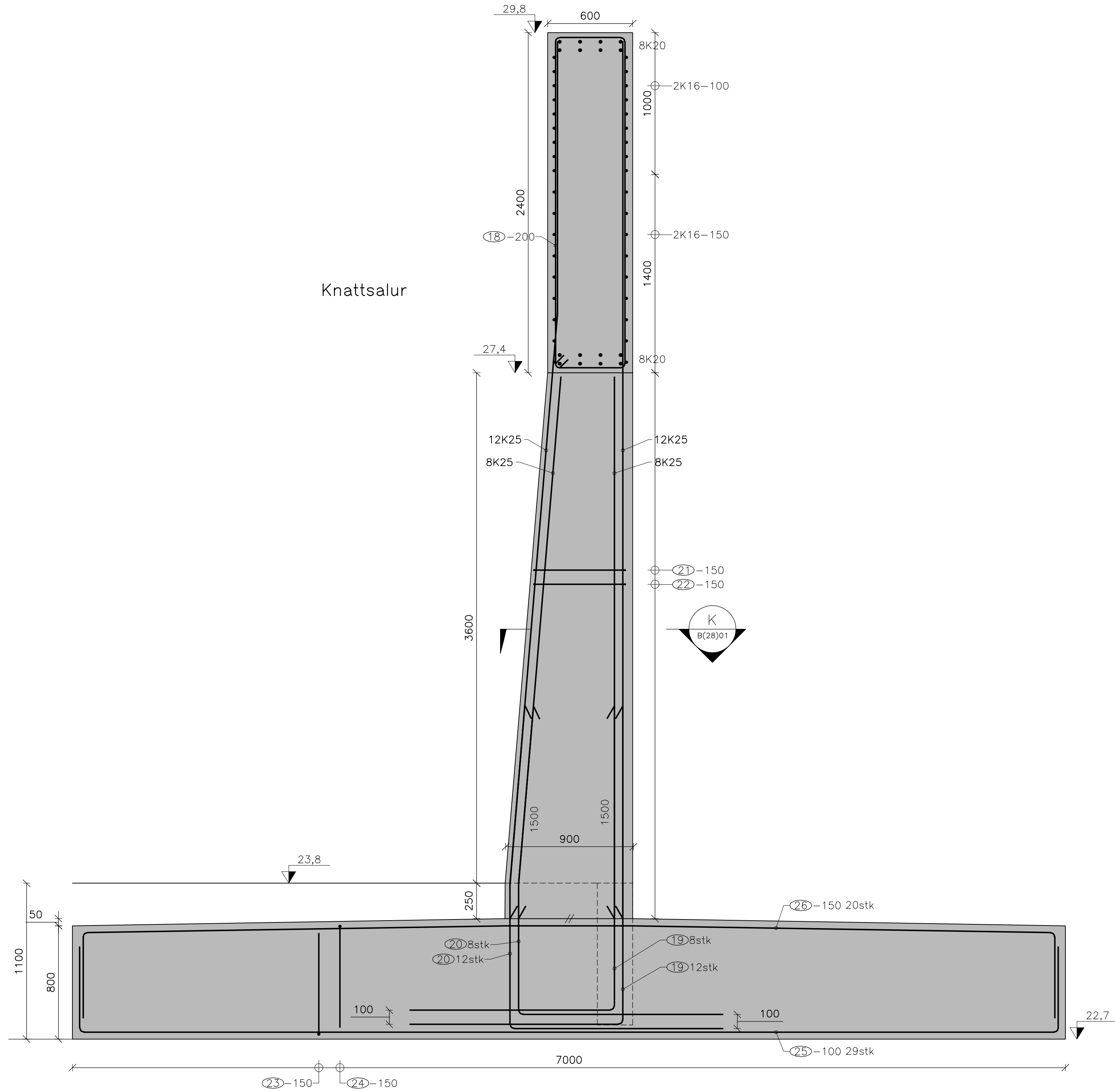
J B(21)07 B(21)08 B(21)09 Súlur i mätlinu 14 Mkv: 1:20
