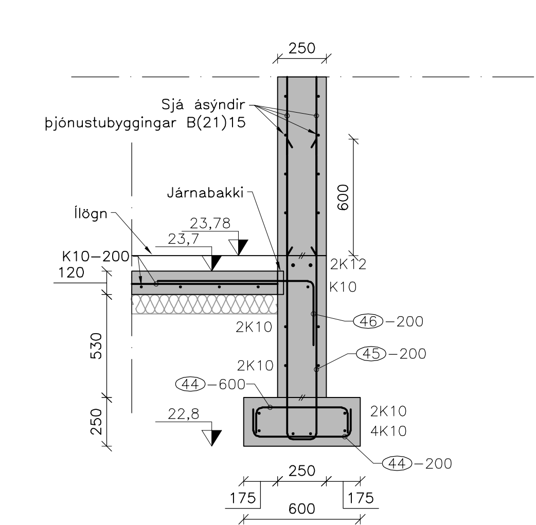
P B(12)02 B(12)03 B(13)01 B(21)15 Snið i sökkul þjónustubyggingar Mkv: 1:20
