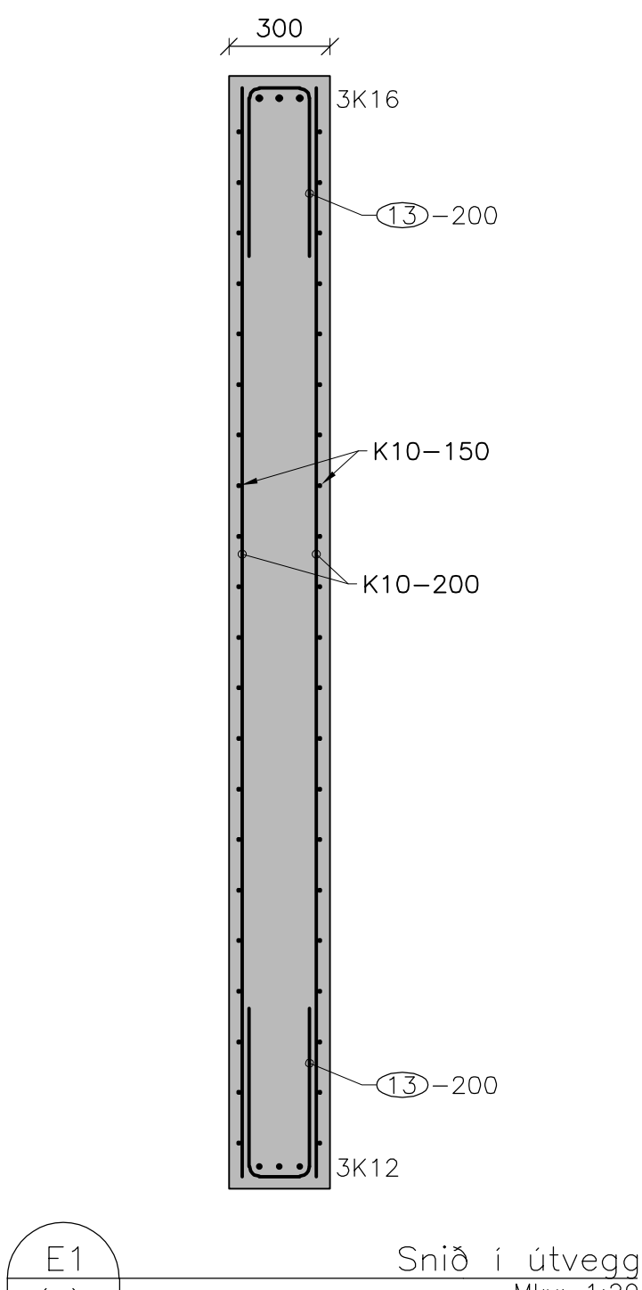
Snið í útvegg Mkv: 1:20
