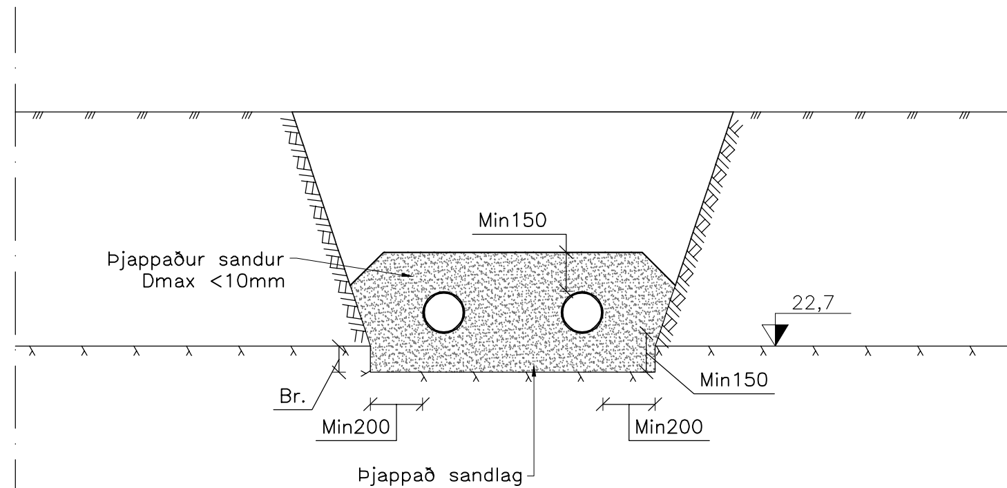
S7 J(11)05 Lagnaskurður Mkv: 1:20
