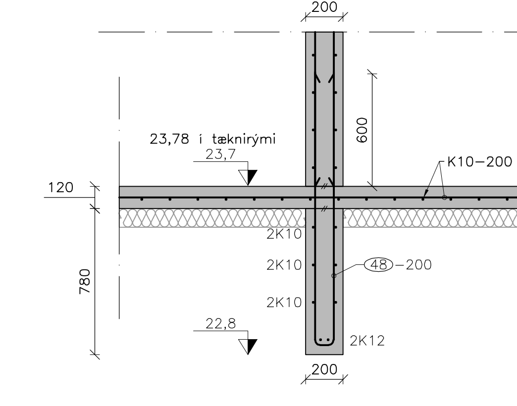
S B(12)02 B(12)03 B(21)17 Snið i sökkul þjónustubyggingar Mkv: 1:20
