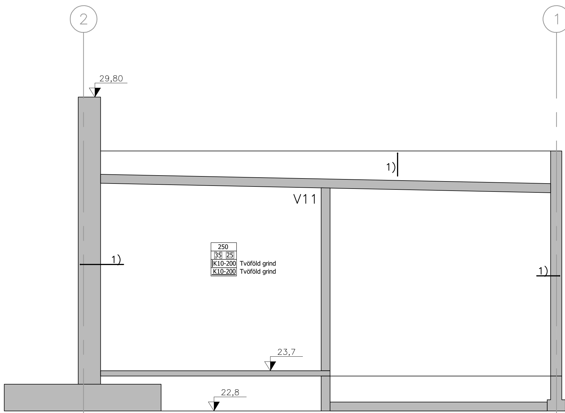
V13 Útveggur þjónustubyggingar í málínu A Mkv: 1:50
