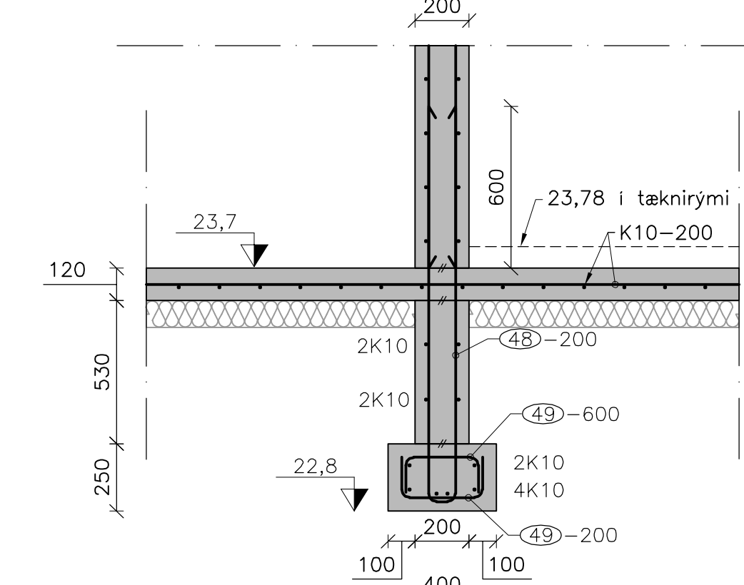
R B(12)02 B(12)03 B(21)17 Snið i sökkul þjónustubyggingar Mkv: 1:20
