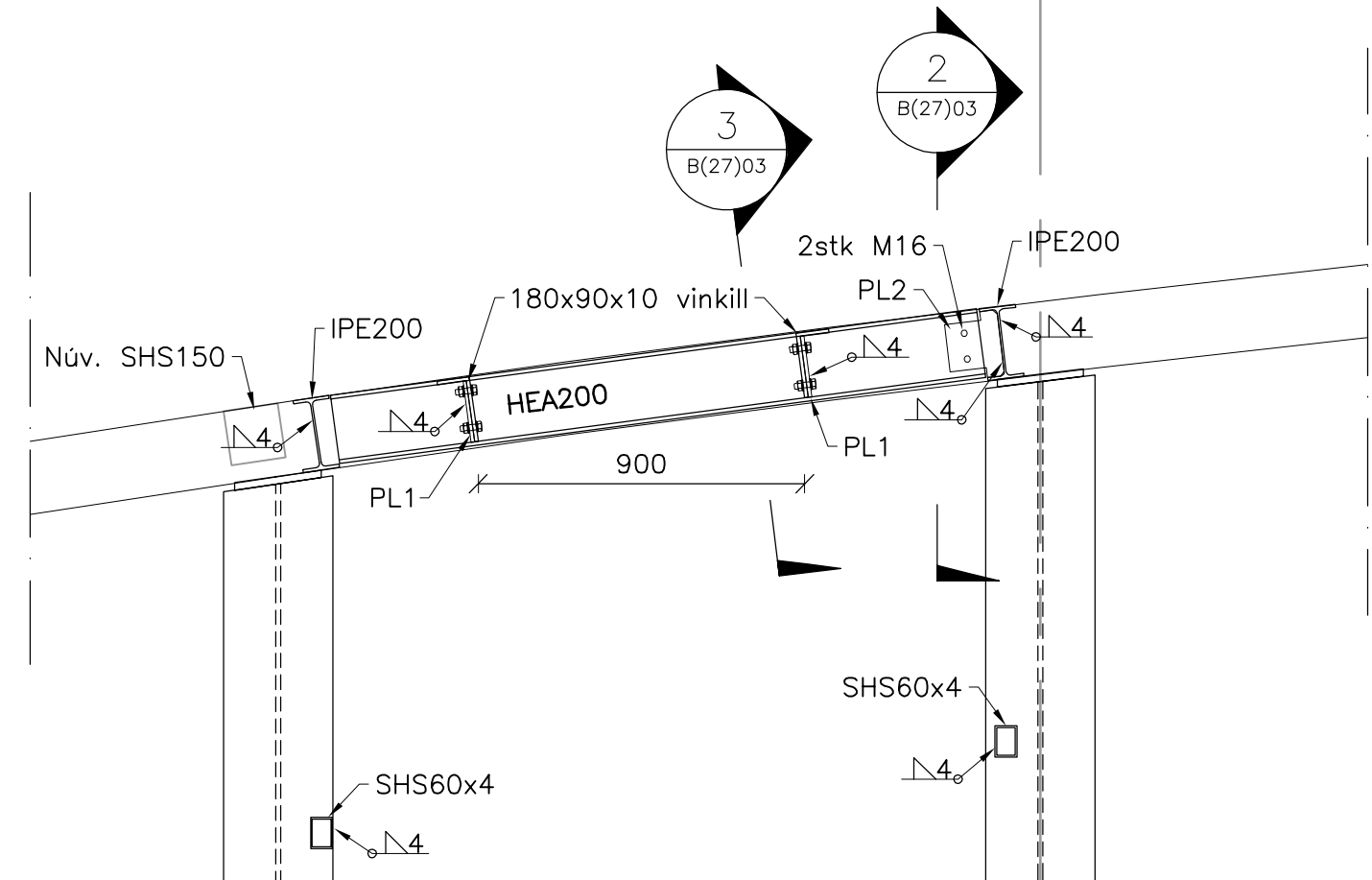
Snið í stál Mkv: 1:20
