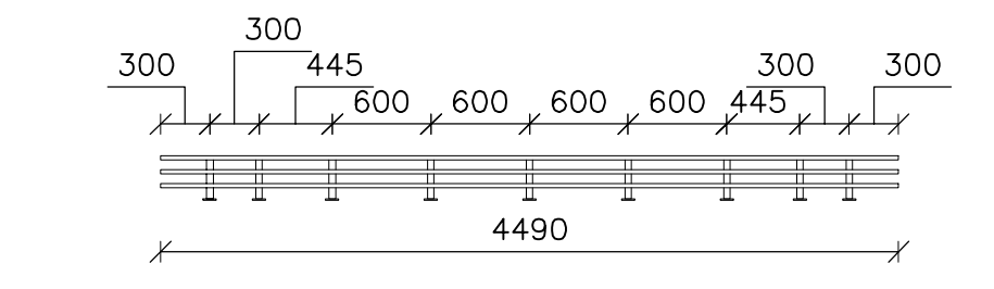
Snjógildra A – 44stk Mkv: 1:50
