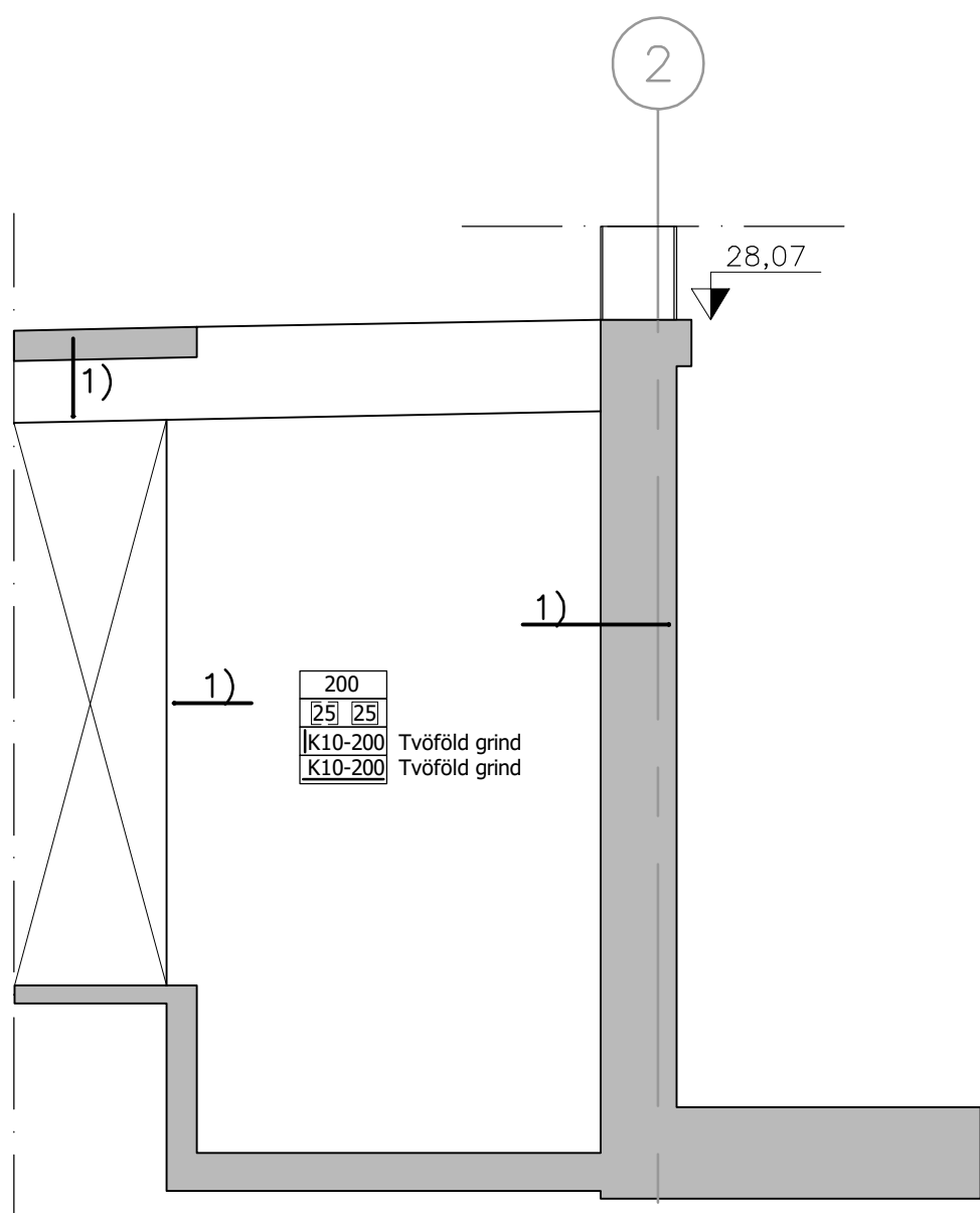
V9 Veggur við lyftugryfju Mkv: 1:50
