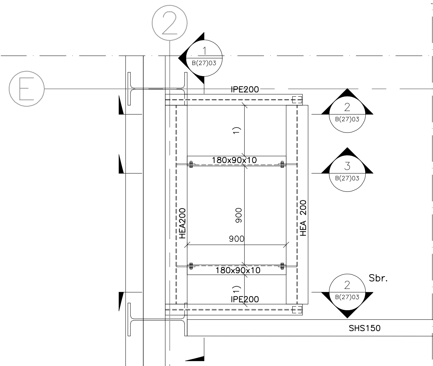
Grunnmynd ops á þaki Mkv: 1:20
