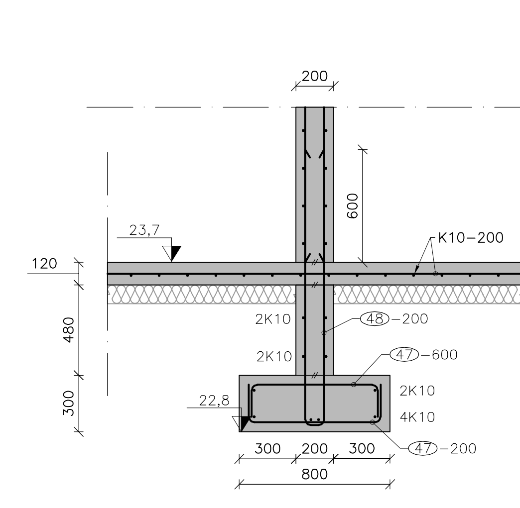
Q B(12)02 B(21)17 Snið i sökkul þjónustubyggingar Mkv: 1:20
