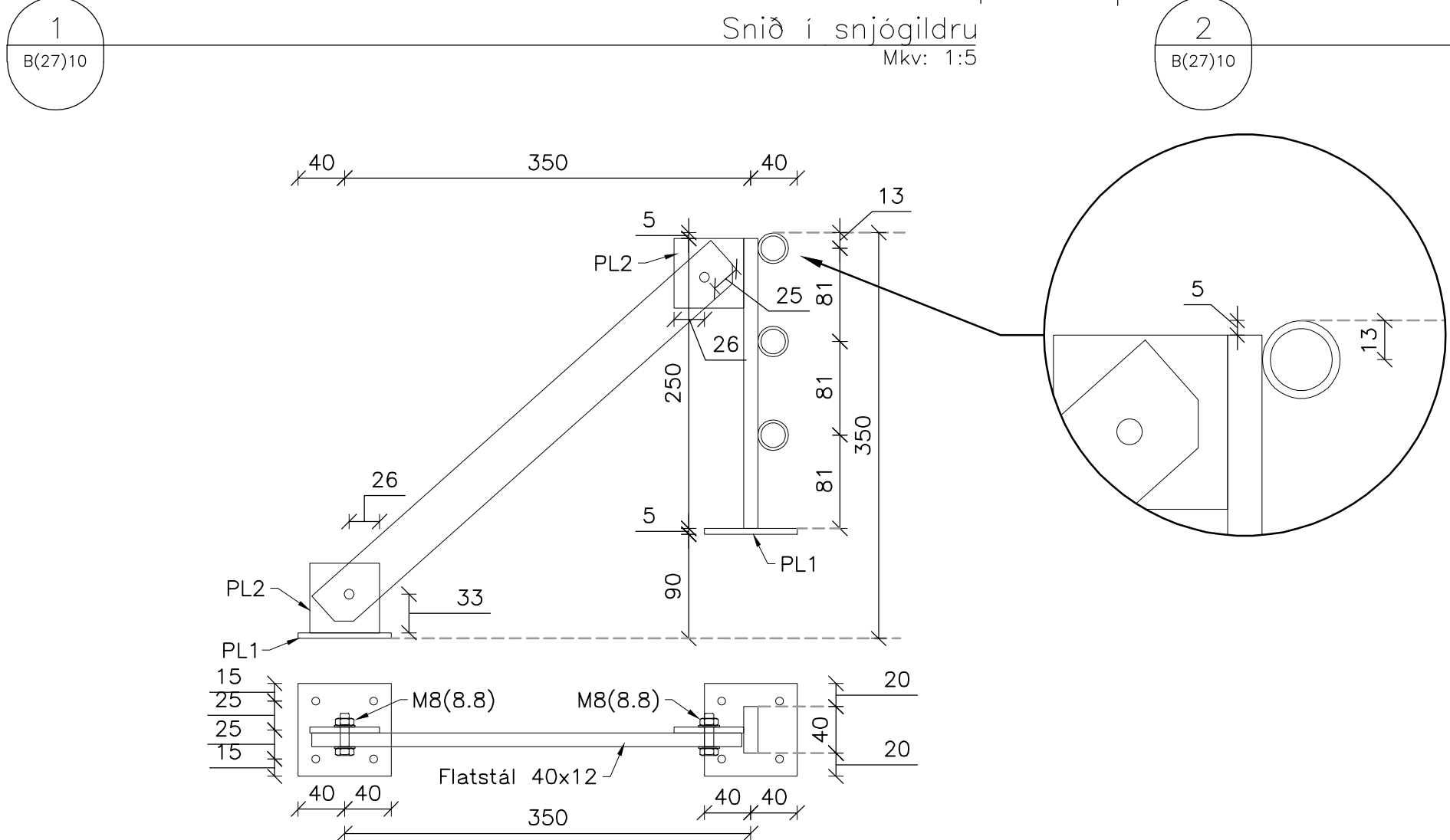
Málsetning stálvinkils Mkv: 1:5
