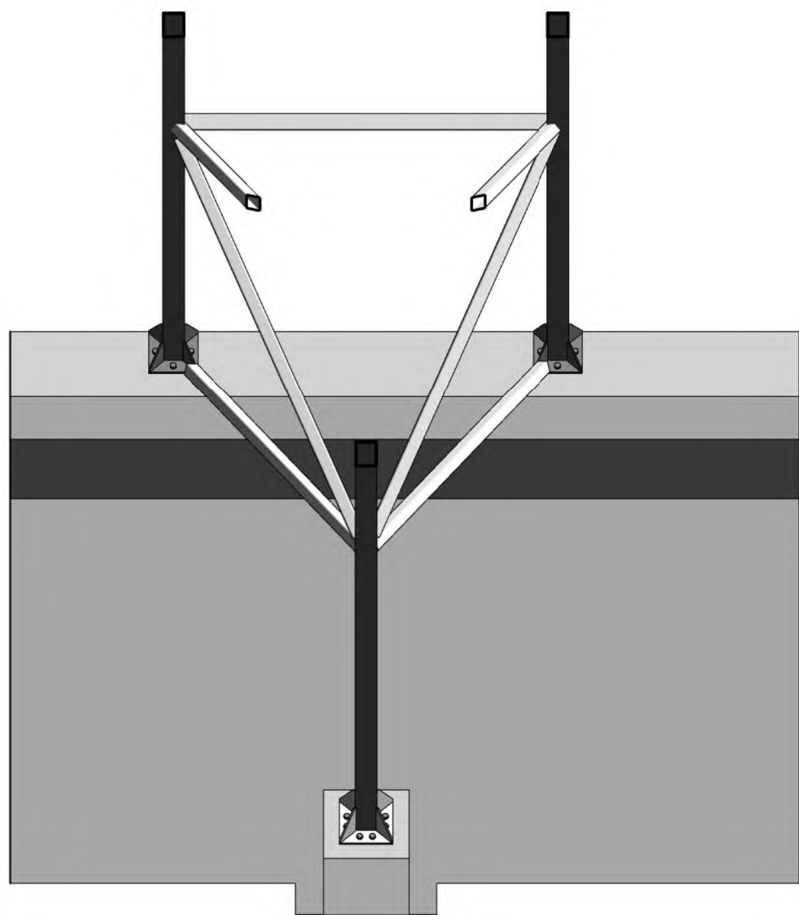
4 Ásýnd á stálboga
