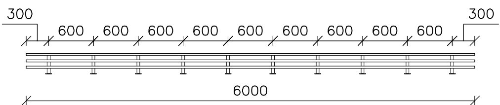
Snjógildra B við gafla – 4stk Mkv: 1:50
