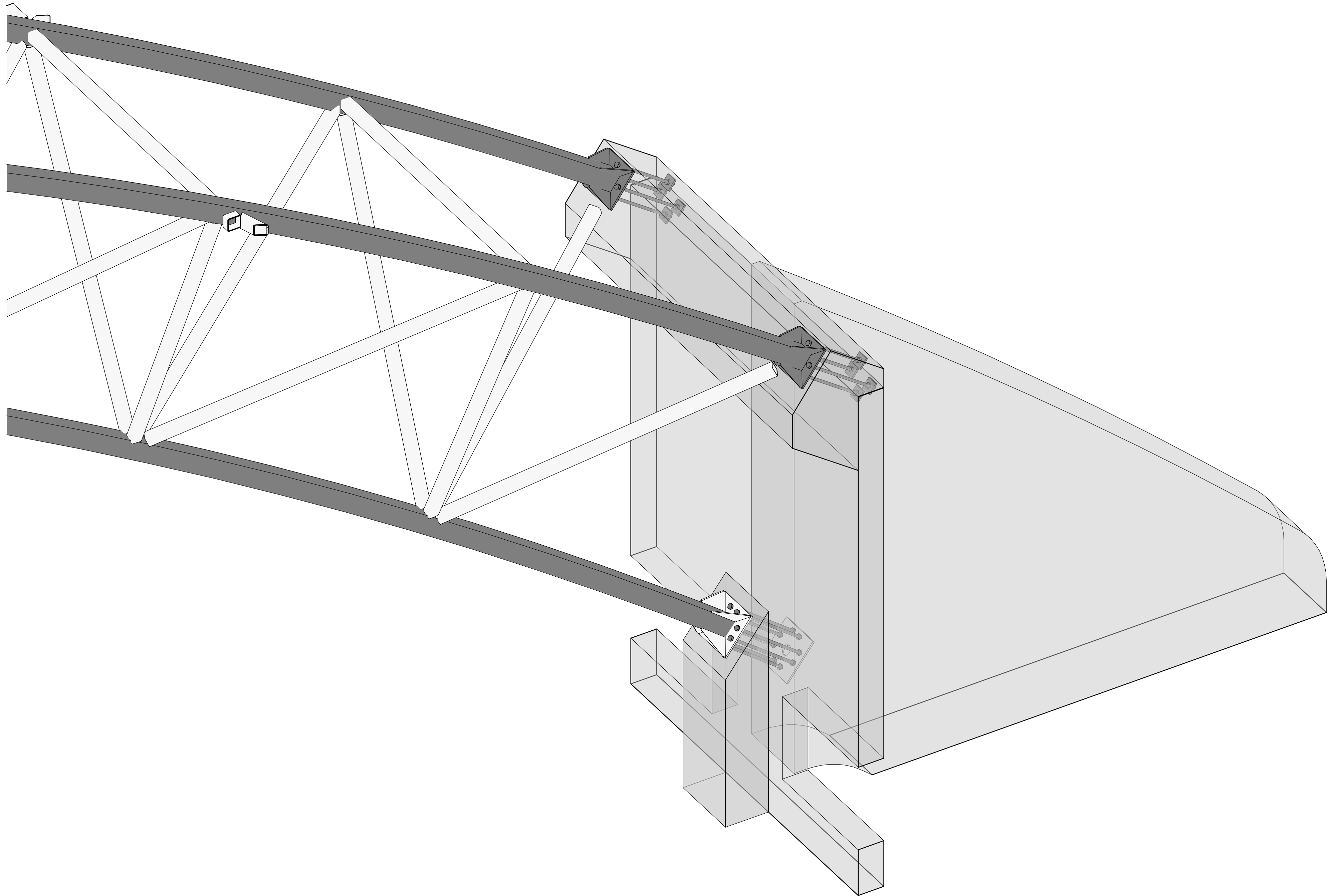
1 3D Steypa og stál
