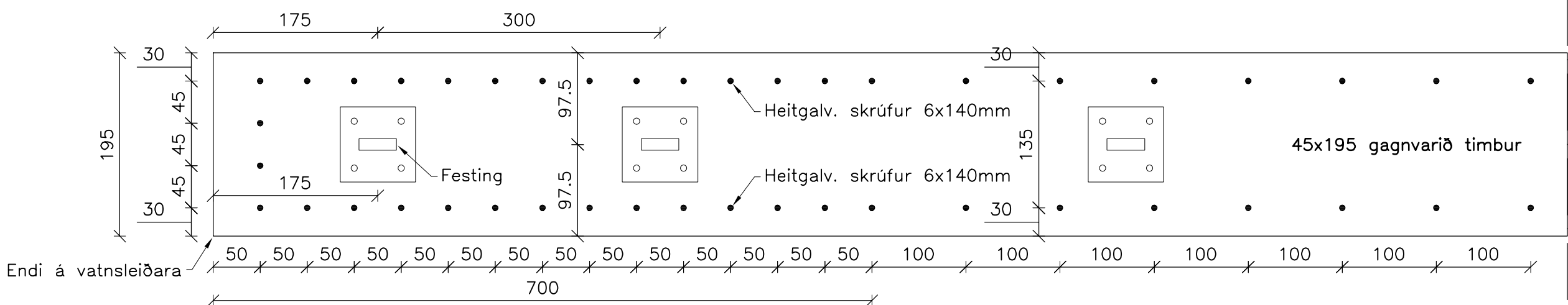
Tréskrúfur í timburreimum / vatnsleiðara Mkv: 1:5
