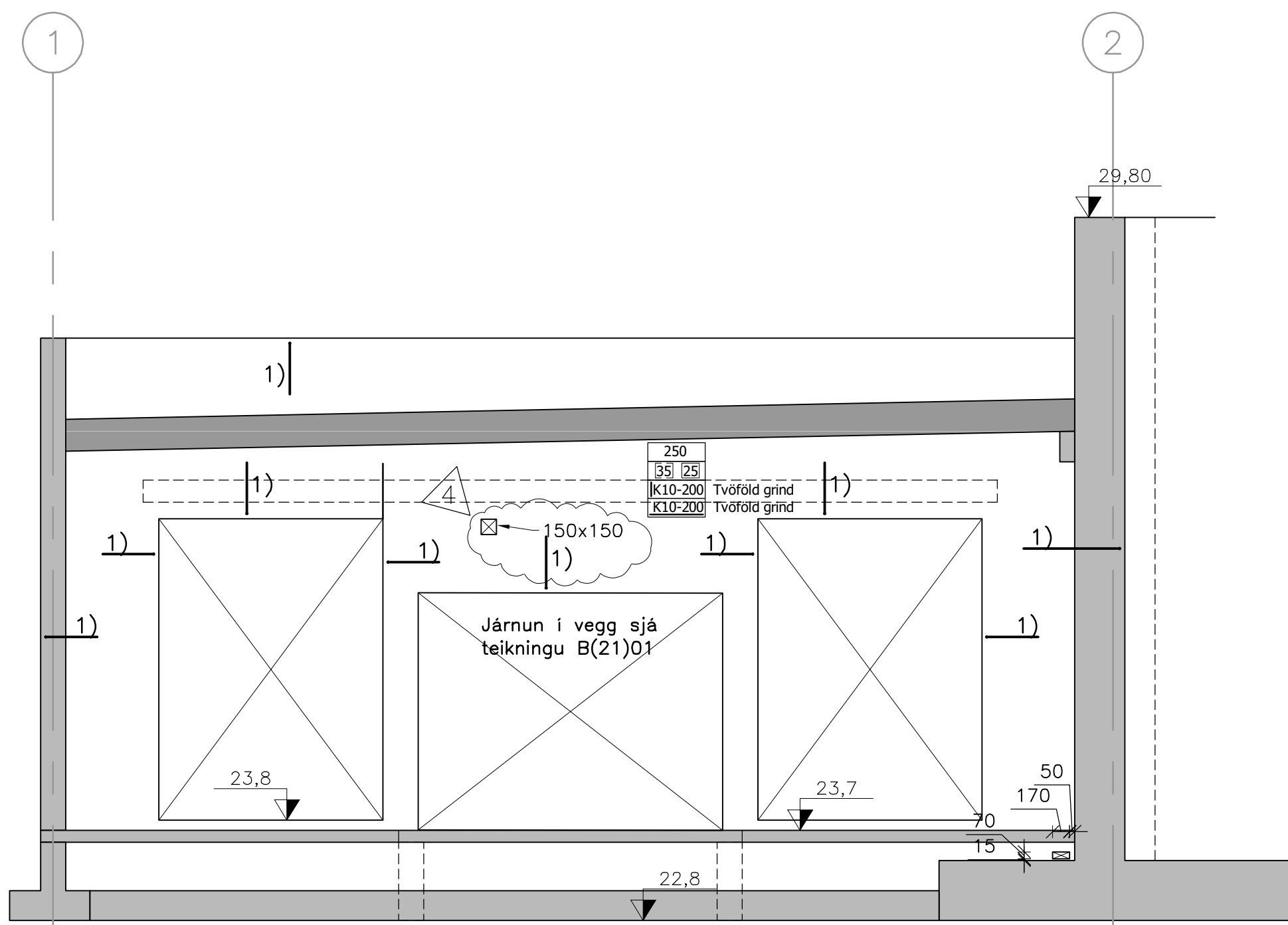
V12 Útveggur þjónustubyggingar í málínu K Mkv: 1:50
