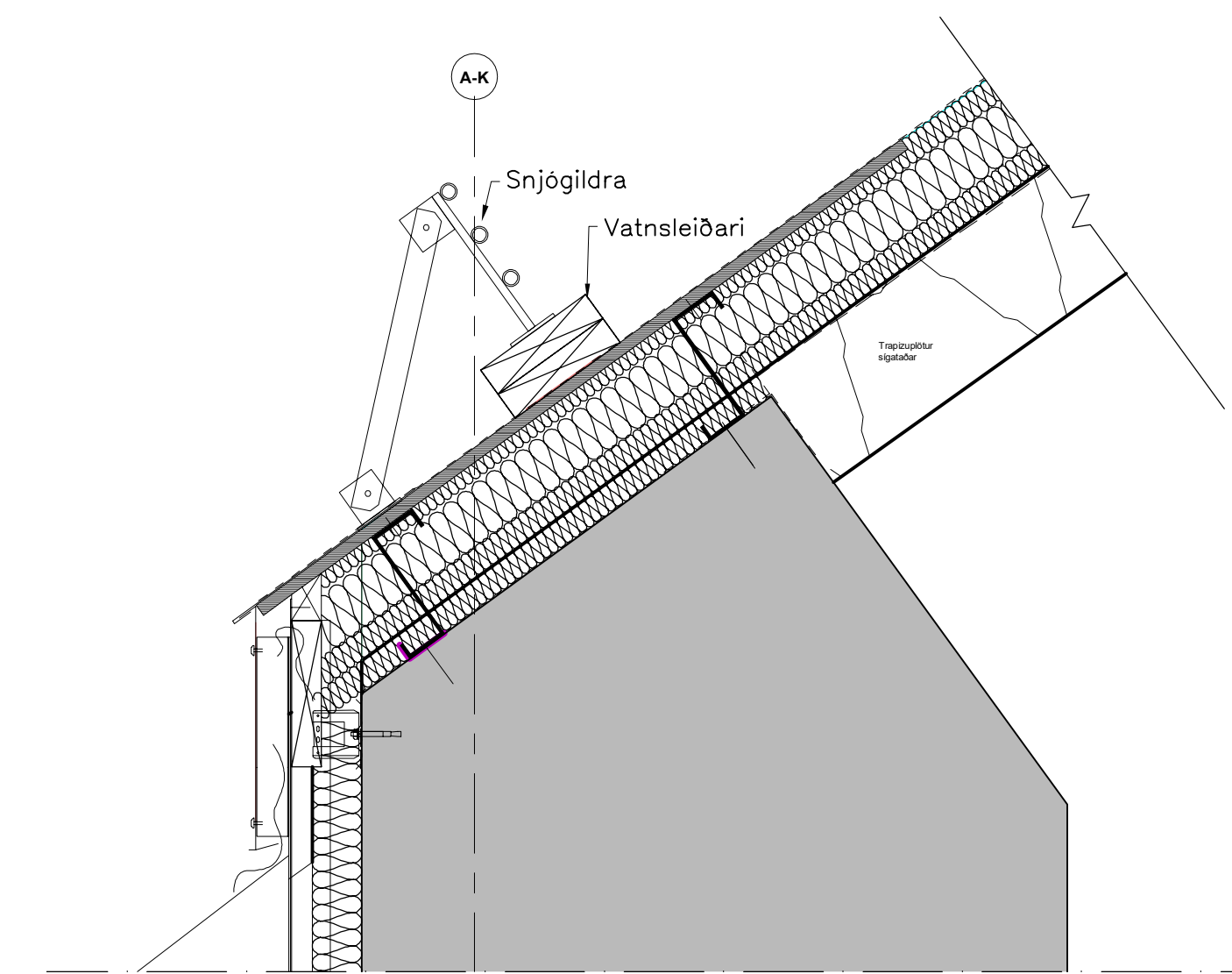
Snið í snjógildru Mkv: 1:10
