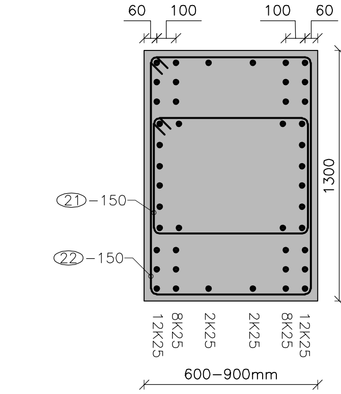
K B(21)07 B(21)08 B(21)09 B(28)01 Snið i súlu i mätlinu 14 Mkv: 1:20
